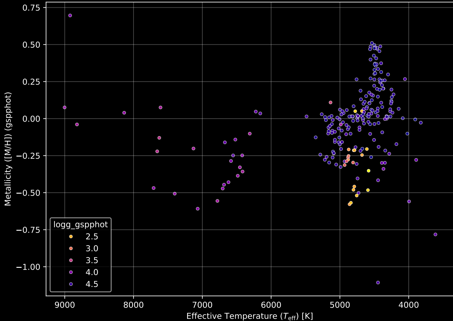
APOGEE DR17 Field: [M67_btx] Stellar Population Parameters (n= 231)
